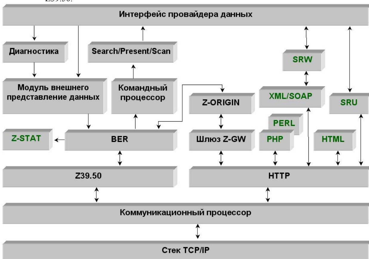
Рис.1. Архитектура сервера ZooPARK v. 5.06
